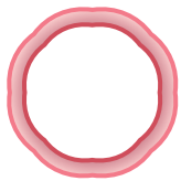
Normal esophagus
